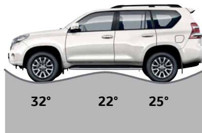
Užvažiavimas, išilginio pravažumo kampas ir nuvažiavimo kampas
